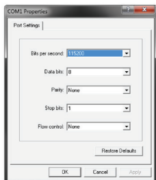
Figure 9. Propriétés de la connexion Hyperterminal
