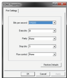
图9. 超级终端连接属性
