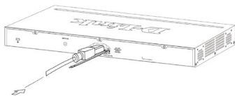
Figura 2-2. Conecte el cable de alimentación al Switch
