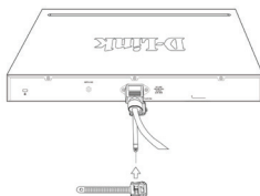
Abbildung 2-3. Kabelhalter durch den Kabelbinder führen
