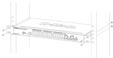
圖 4. 安裝交換器到標準尺寸的機架
