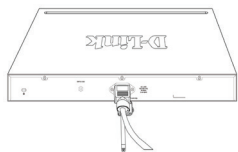
Figura 2-5. Asegurar el cable de alimentación
