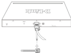
Gambar 2-3. Geser penahan melalui "Tie Wrap"
