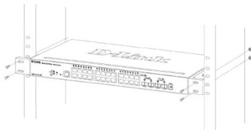
Gambar 4. Memasang switch ke rak dengan ukuran standar
