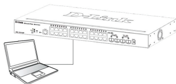
Рисунок 6. Подключение Ethernet-кабеля
