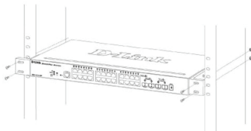
Figura 4. Instalando o switch em um rack de equipamentos tamanho padrão
