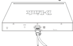
Abbildung 2-5. Stromkabel sicher befestigen
