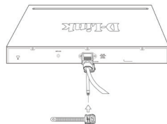
Figura 2-3. Deslize o retentor através da braçadeira
