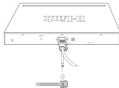
Figura 2-3. Deslice el retenedor a través de la banda de sujeción
