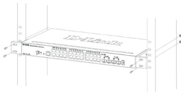
图 4. 安装交换机到标准尺寸的机架
