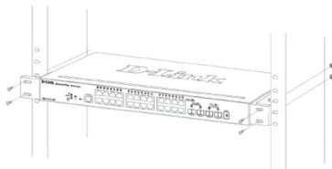
Figura 4. Installazione dello switch all'interno del rack
