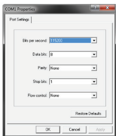
Figura 9. Propiedades de la conexión de Hypertterminal
